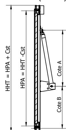
B-B ( 1:16 )
